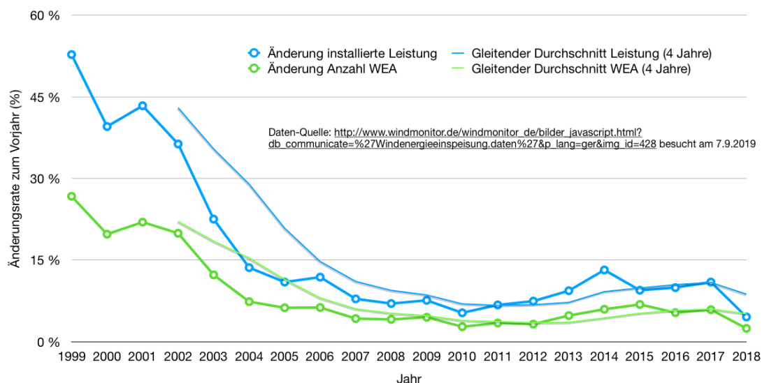
Abbildung 1 - Verlauf des Zubaus von WEA 1999-2018
